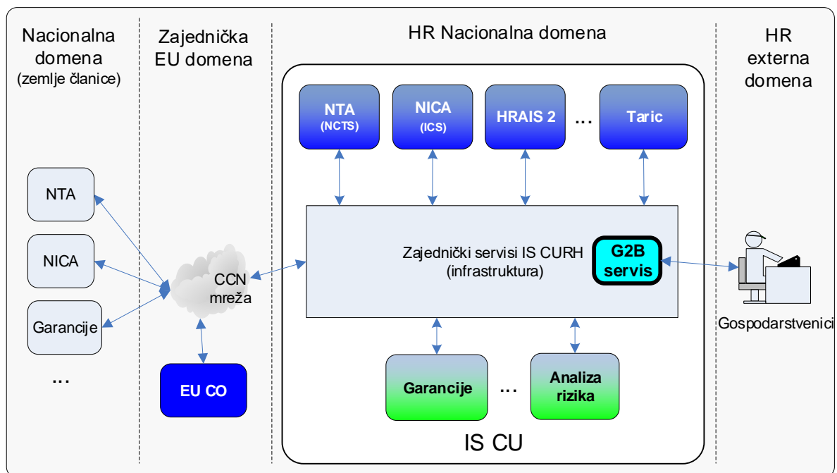
Slika 1 Koncept arhitekture
